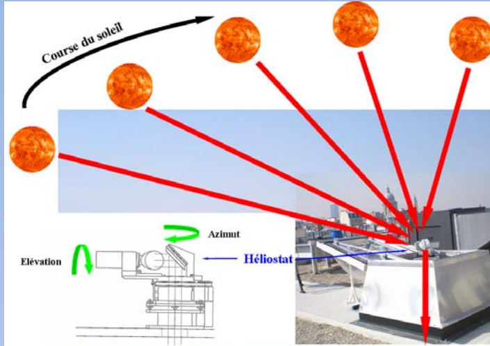
L'héliostat
